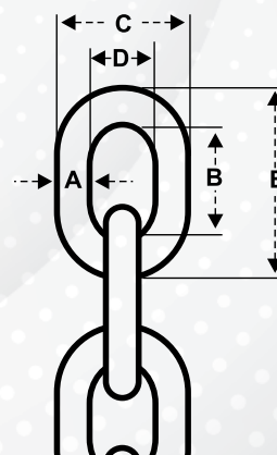
Διαστάσεις (mm)
